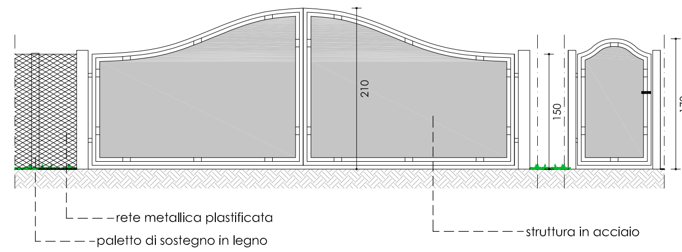
PROSPETTO ACCESSO CARRAIO E PEDONALE "1" - scala 1:50
