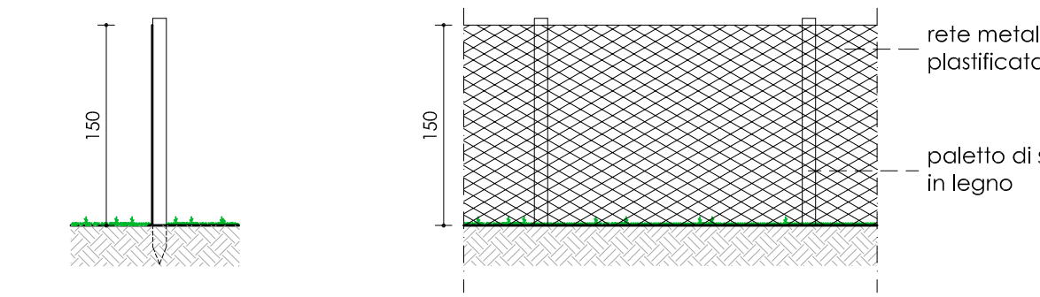
SEZIONE A-A - scala 1:50
