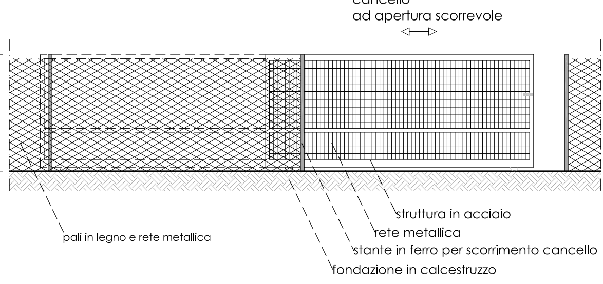
PROSPETTO ACCESSO CARRAIO "3" - scala 1:50
