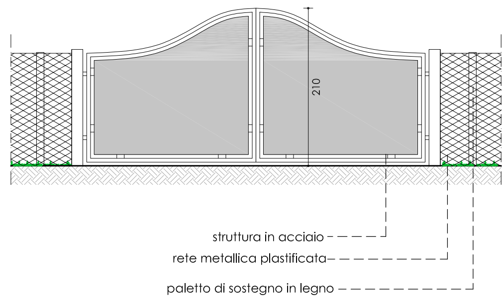
PROSPETTO ACCESSO CARRAIO "2" - scala 1:50
